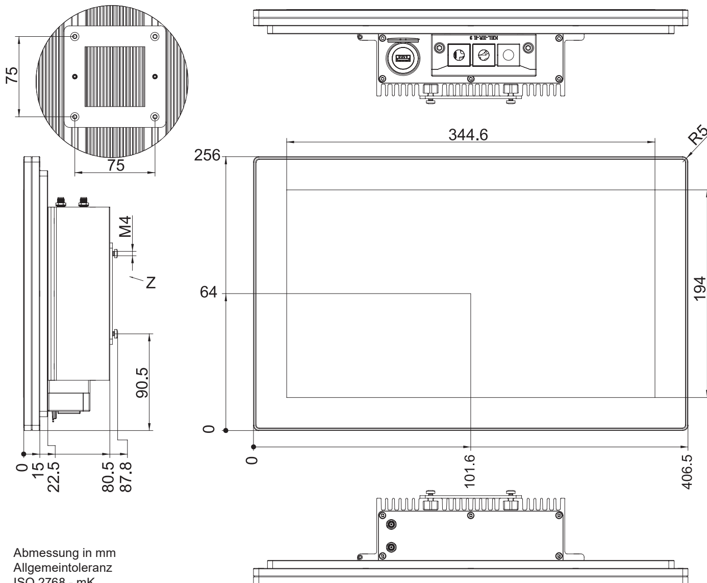
Ansicht Z / View Z
