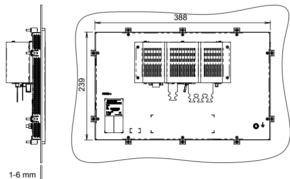
Montage / Einbauausschnitt Assembly / Installation cut-out
